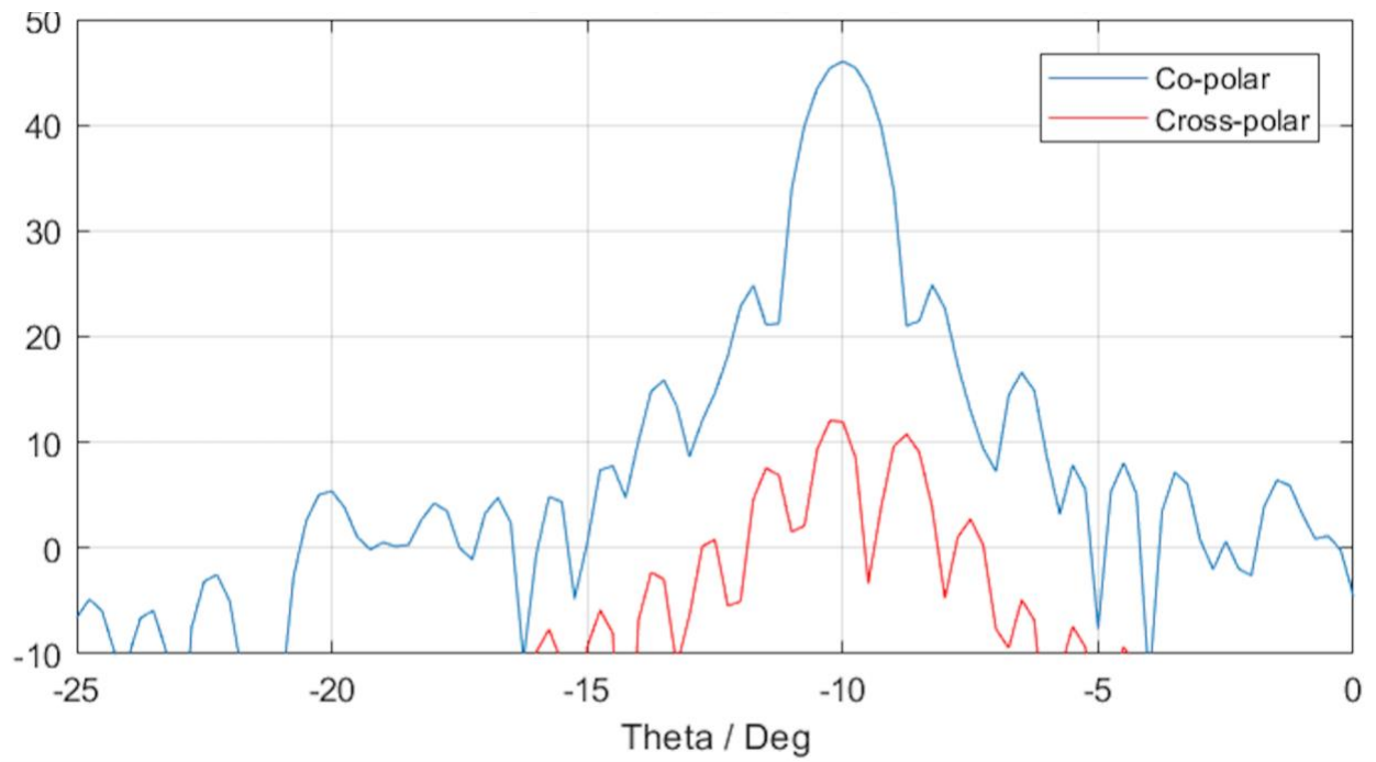
Radar Antenna H-plane
