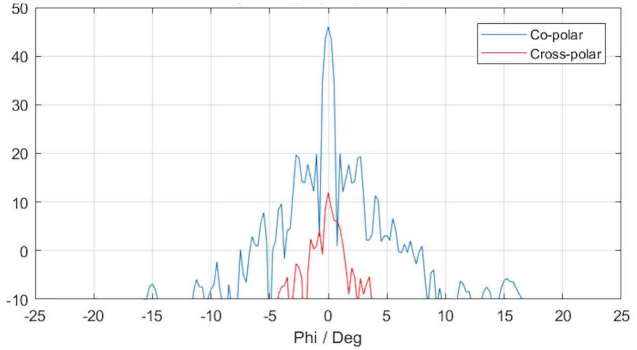
Radar Antenna V-plane
